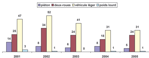
Accidents corporels de la circulation routière 2001 - 2005
